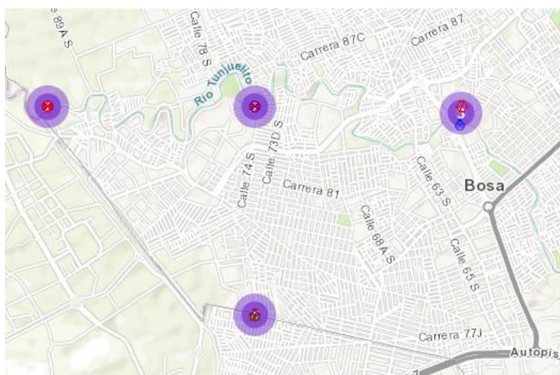
Figura N° 3. Estaciones Meteorológicas aledañas a la localidad de Bosa
